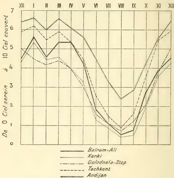
Fig. 3. — Nébulosité moyenne dans quelques stations du Turkestan russe.
