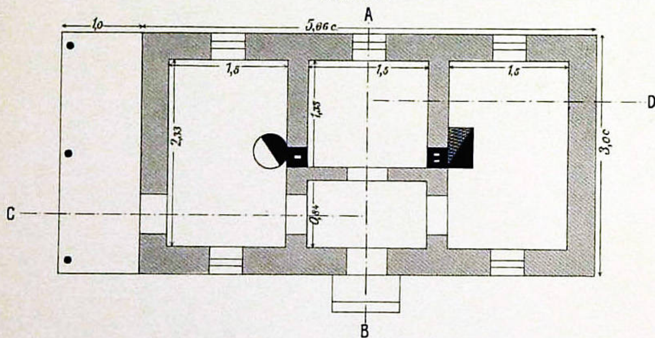
Планъ
