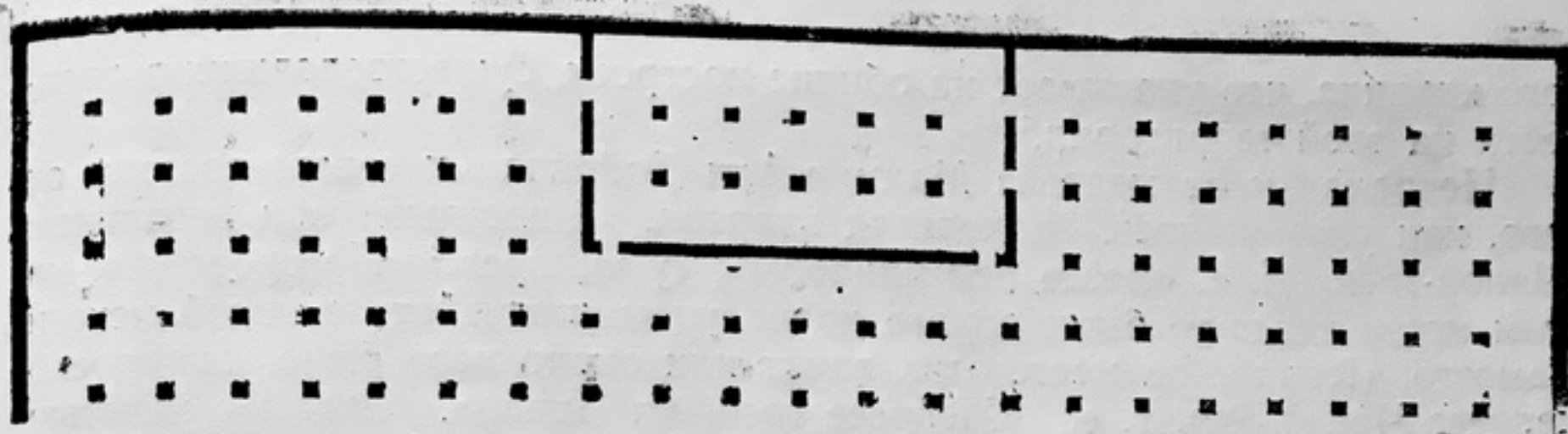
Рис. 8. Схема плана кокандской соборной мечети, построенной в первой четверти XIX в.
