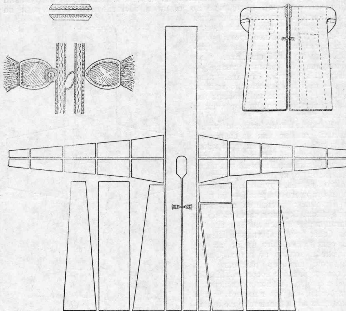
Рис. 13. Покрой фаранҷи.
