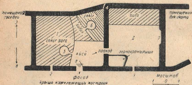
Рис. 19. Жилище Джума Одина в сел. Деги-балайд. I — mūr ; II — kánpa ; 1 — дверь; 2—4 — окна; 5—6 — очаги; 7 — ниша; 8 — лестница из каменных плит.
