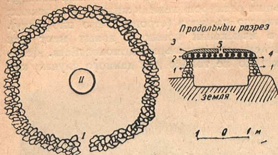
Рис. 30. План „дома для гостей“, летовка Куливорсоут. 1—стена каменной кладки; 2—жерди; 3—слой щебня и земли; 4—балки; 5—отверстие для выхода дыма; I—проход; II—место для костра.
