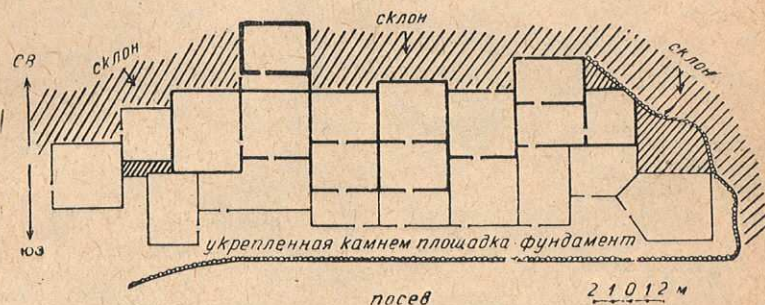
Рис. 14. План многосемейного жилища-квартала в сел. Кули-миона. Острая линия — первый этаж (хлевы); полу жирная линия — второй этаж (жилые помещения); жирная линия — третий этаж (дом для гостей); линия из точек — стена каменной кладки для защиты от завала снега.
