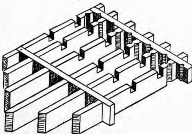
Рис. 132. Сборка наборных решеток.
