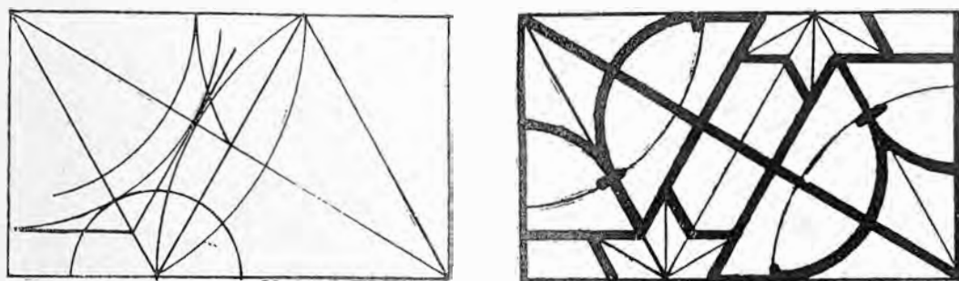
Рис. 93. Схема построения элементов решетки № 48.
