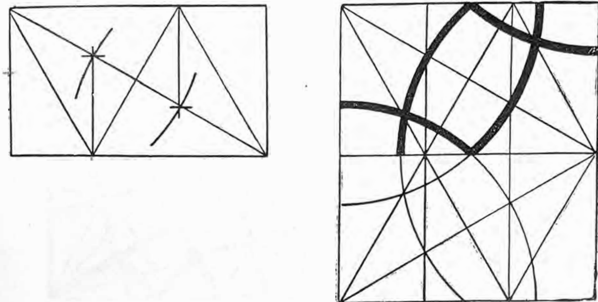
Рис. 82. Схема построения элементов решетки № 43.
