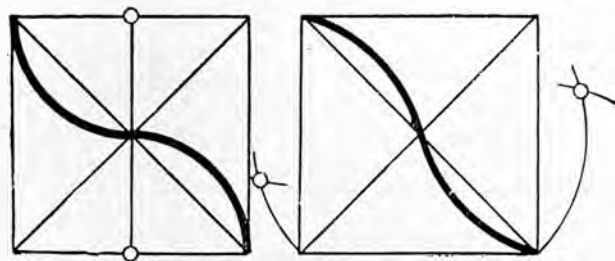
Рис. 121. Схема построения кривых: а) каблук, б) гусёк.
