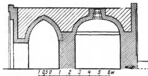
Рис. 10. Поперечный разрез
