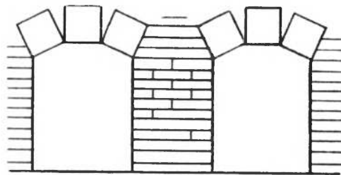
Рис. 14. Устройство забулки сводов галереи
