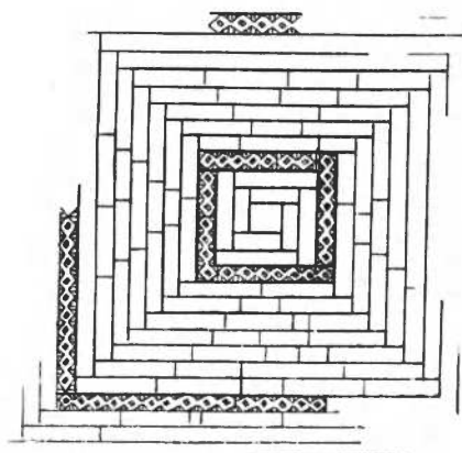
Рис. 7. Замок свода «балхи»
