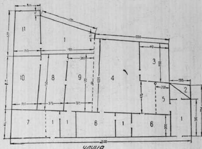
Khiva. Plan schématique d'une maison d'habitation
