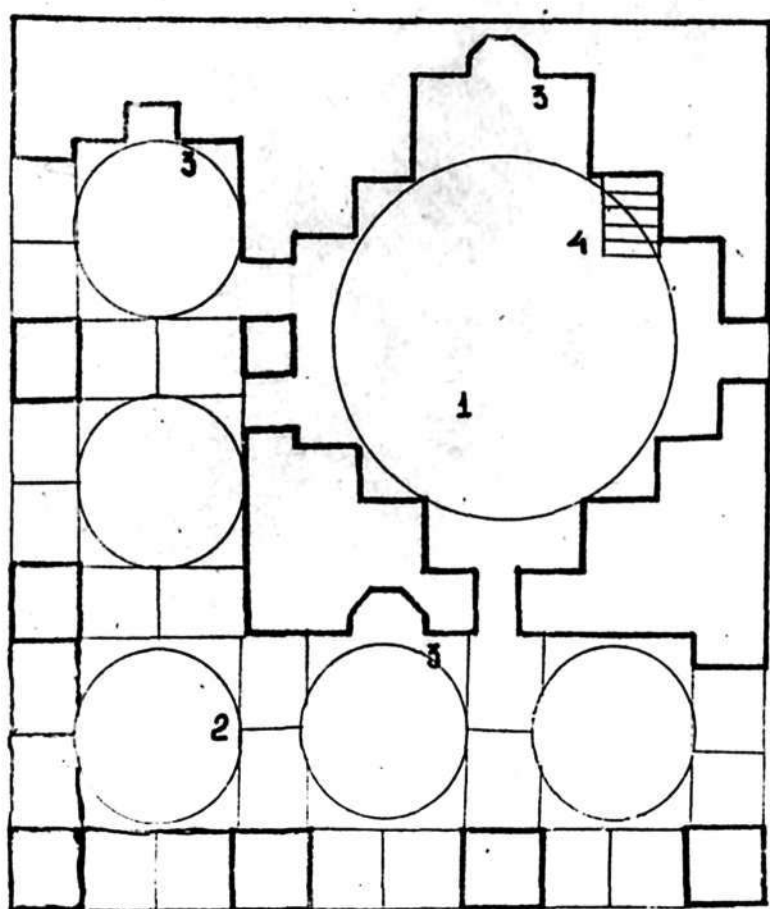
Рис.3. План и разрез Мачити Сангина
