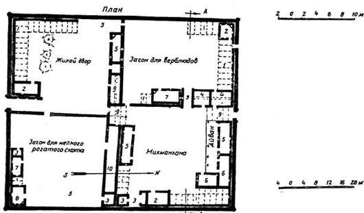
Рис. 50. Кувакский район. Ховлы Баба Нарзабая. План участка и разрез 1 — навес для лошадей; 2 — зимунчик; 3 — хозяйственный склад; 4 — амбар; 5 — жилое помещение хозяев; 6 — жилое помещение для гостей; 7 — жилое помещение для пастухов; 8 — маслобойка; 9 — крытый проход; 10 — коровник
