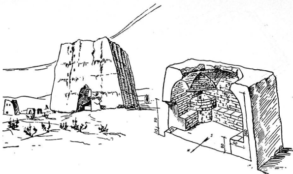
Рис. 17. Анау. Руины дома и детали конструкции перекрытия
