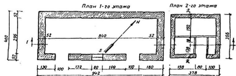
Рис. 47. Астана-Баба. Ховлы Джума Джебарова. Жилые постройки
