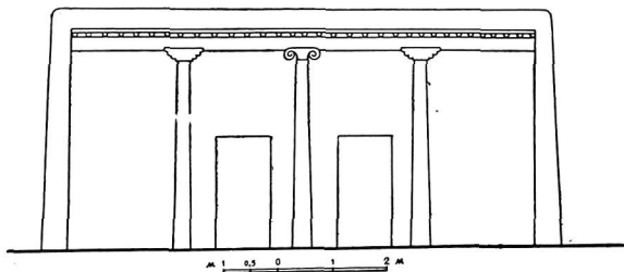
Рис. 7. С. Мурча. Мечеть. Разрез
