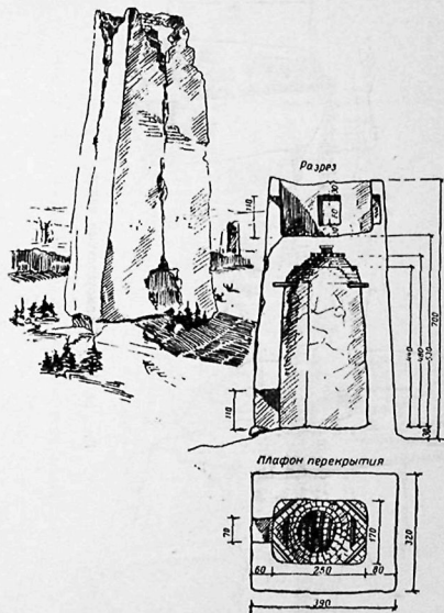
Рис. 13. Анау. Динг (башня). Разрез и конструкция перекрытия
