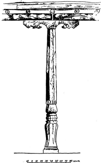
Рис. 44. Район Лямбе. Колонна айвана
