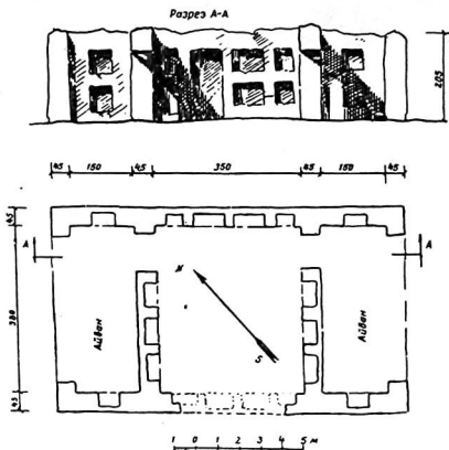
Рис. 21. Пештак. План и разрез жилого дома
