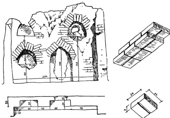
Рис. 18. Анау. Детали оформления стен интерьера. Приемы сырцової кладки
