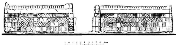
Рис. 34. Район Саккара. Фасад усадьбы
