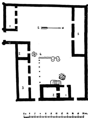
Рис. 30. Район Кагановическа. План усадьбы
