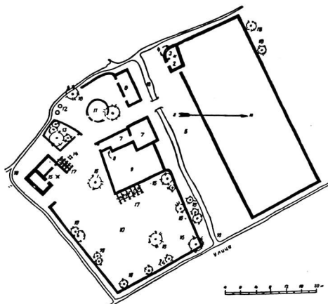
Рис. 49. Астана-Баба. Ховлы Джама Джабарова. План участка 1 — посевы пшеницы; 2 — открытый дворик; 3 — навес; 4 — продукты на уровне земли; 5 — проезд между приусадебными постройками; 6 — жилое зимнее помещение; 7 — склад топлива и хозяйственного инвентаря; 8 — окно-лаз; 9 — посев лука и моркови; 10 — посев джугары; 11 — летнее жилое помещение (юрта); 12 — очаг и тандыр; 13 — загон для скота; 14 — колодец; 15 — жилое зимнее помещение с айваном и саманханой; 16 — древесные насаждения; 17 — виноградник; 18 — арык
