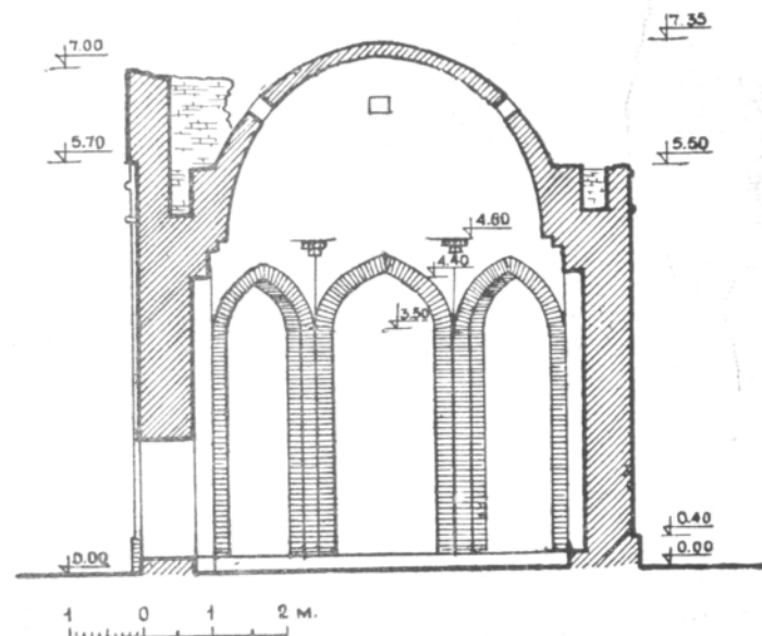
Рис. 85. Мавзолей Кара-Куль. Разрез.
