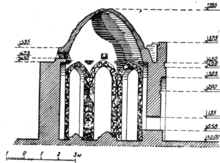
Рис. 64. Мавзолей Торг-Кара. Разрез.
