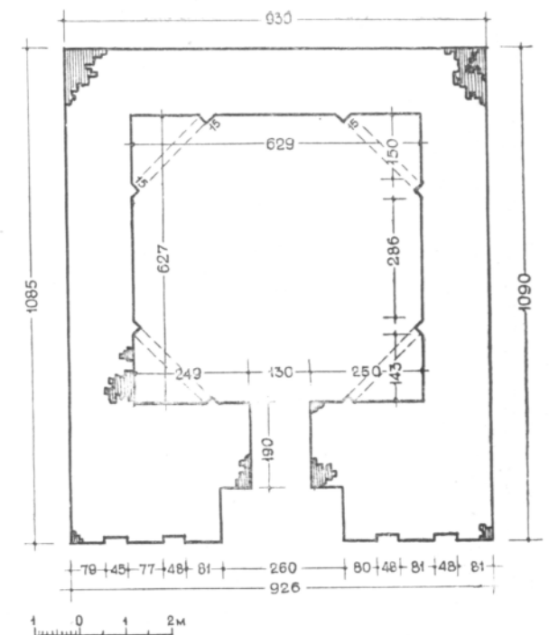
Рис. 39. Мавзолей Болган-ана. План.
