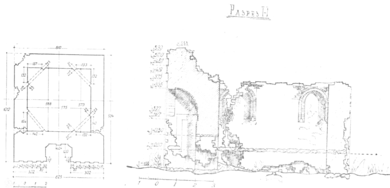
Рис. 11. Мавзолей Аяк-Хамыр. План на отметке 4; 3,20,
