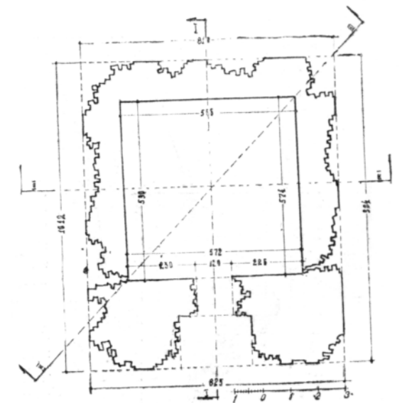
Рис. 9. Мавзолей Аяк-Хамыр. План на отметке \sim 0,00 .
