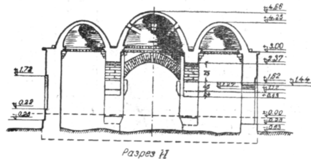
Рис. 79. Мавзолей Косубай-Кара. Разрез.
