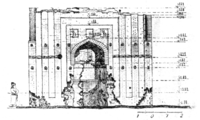
Рис. 7 .Мавзолей Аяк-Хамыр. Главный фасад.
