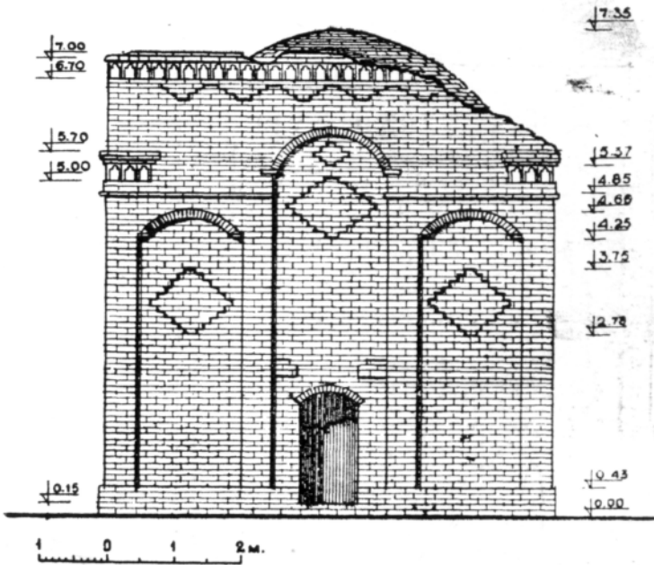
Рис. 82. Мавзолей Кара-Куль. Главный фасад.
