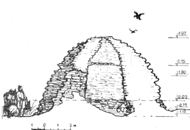
Рис. 3. Маазолей Домбаул. Разрез.
