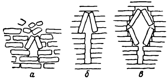
Рис. 3. Формы бойниц
