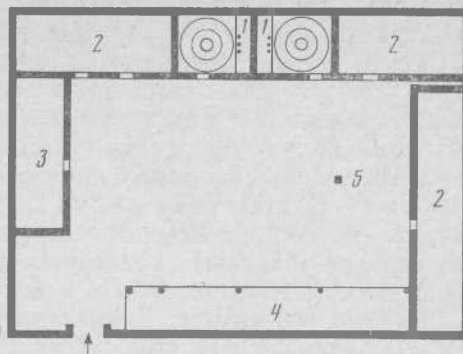
Рис. 4. Маслобойня (джувозхона) в Хуфаре: 1 — собственно джувозхона, 2 — стойло для быков ( гаухона ), 3 — стойло для лошадей ( аспхона ), 4 — навес с кормушками ( чуптора ), 5 — привязь для лошади ( яккамех )
