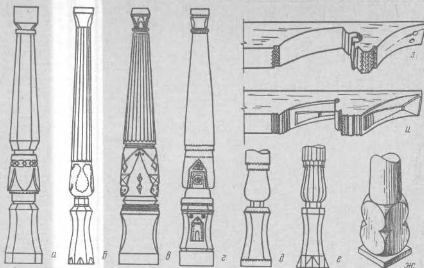
Рис. 5. Колонны Сурхандарьинской области: а — в мечети Суфи Алласта в Катта Вахшуваре, б — в мечети Дашнабада, в, г, д — в мечети Лючико в Хуфаре, е, ж — в мечети Мирзоб в Хуфаре; подбалки: з — в мечети Дашнабада, и — в мечети Лючико в Хуфаре
