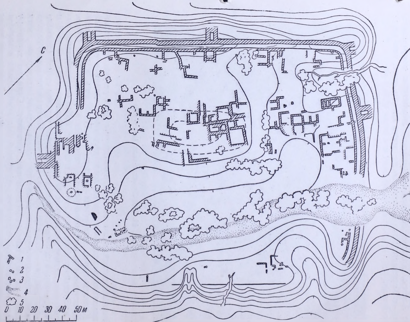
Рис. 13. Қанга-кала (план крепости): 1 — выходы стен; 2 — хумы; 3 — плиты (известняк); 4 — песчаная гряда; 5 — кустарник
