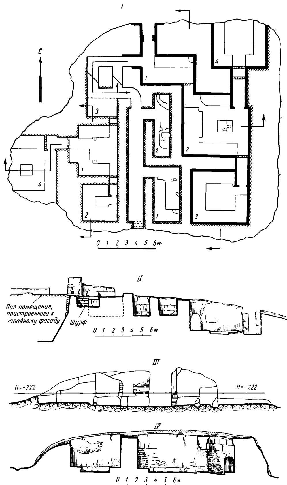
Рис. 2. Городище Кахкаха II. План и разрезы замка последней реконструкции I — план; II — разрез З — В (вид на север); III — разрез Ю — С по верхнему ярусу (вид на запад); IV — разрез Ю — С по нижнему ярусу (вид на запад)
