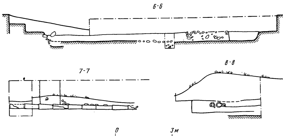
Рис. 2. Архитектурные разрезы
