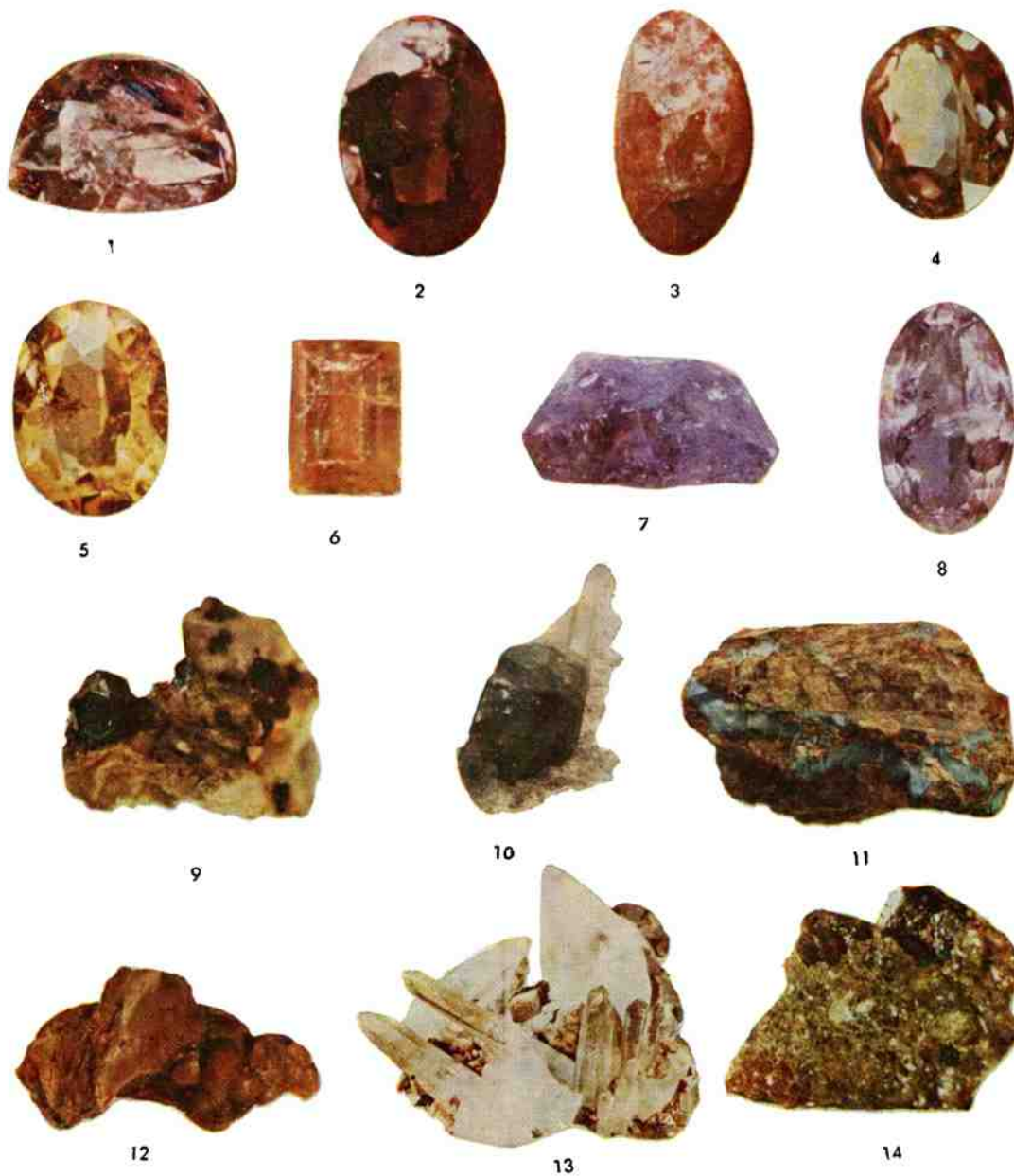
Ограночные камни. 1—4. Бадахшанские далы (благородная шпинель). 5—6. Клиногумит. 7—8. Аметист. 9—10. Кристаллы турмалина в породах. 11. Пржилки бирюзы в песчанике. 12. Сердолик. 13. Друза горного хрусталя. 14. Кристаллы граната в породе.
