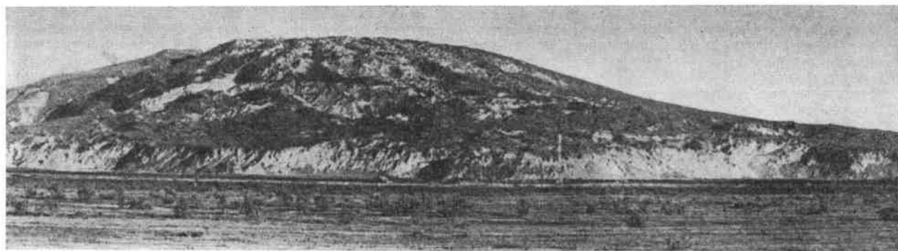
Соляной купол Ходжамунин.
